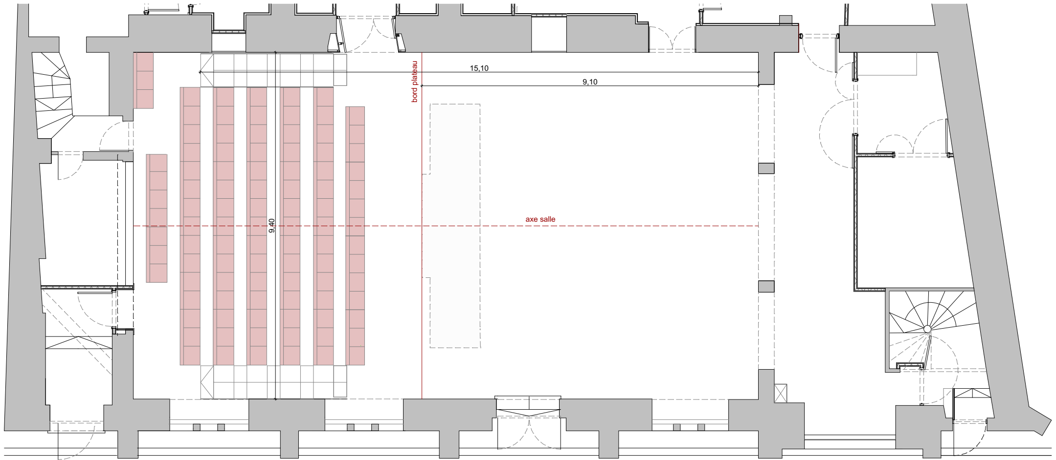
TJP PETITE SCENE VUE EN PLAN ECHELLE 1/100 GRADIN DEPLIE - FOSSE FERMEE
