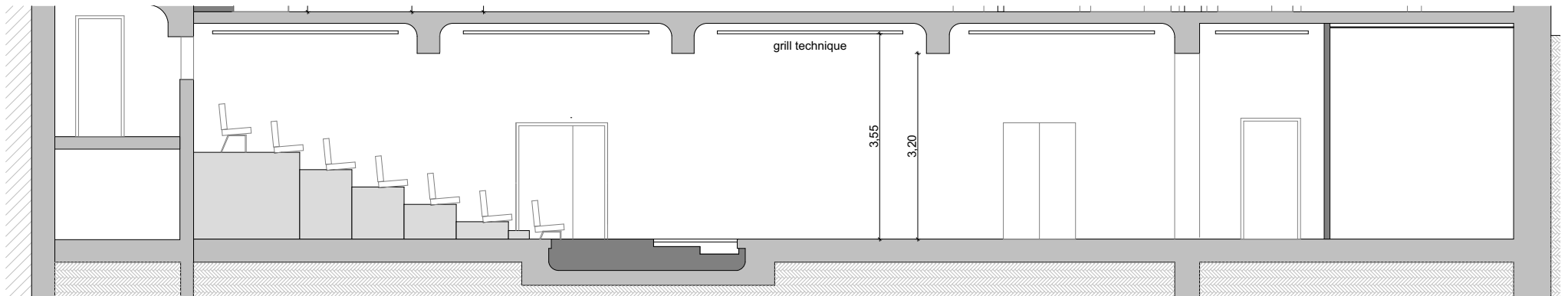
TJP PETITE SCENE COUPE LONGITUDINALE ECHELLE 1/100
